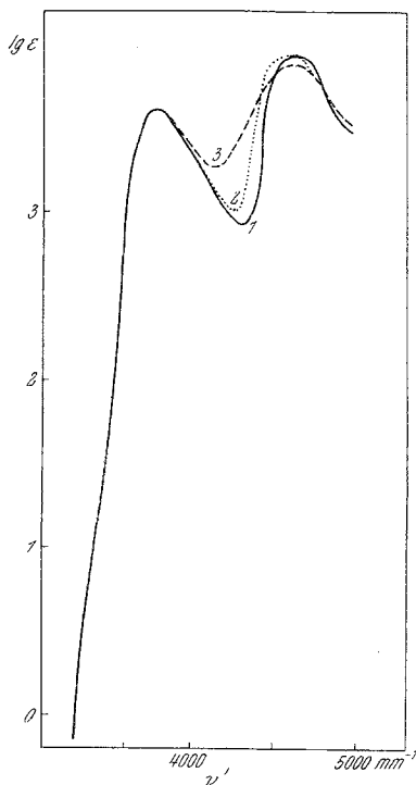
Abb. 4. UV-Spektrum von \alpha -Cyanpyridin 1 in 0,05 n HCl; 2 in \text{H}_2\text{O} ; 3 in 0,05 n NaOH
