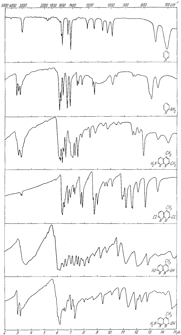
Abb. 5. UR-Spektren einiger Pyridine und Naphthyridine
