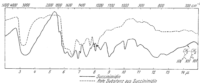
Abb. 2. UR-Spektren von Succinimidin (—) und der daraus erhaltenen roten Substanz (---)
