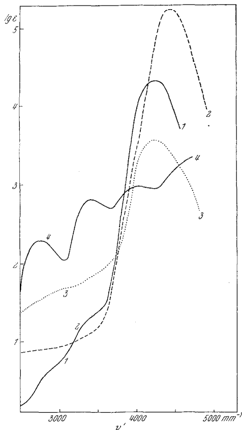
Abb. 1. UV-Spektren von: 1 Succinimidin in Äthanol 2 5-Imino-2-pyrrolidon in Äthanol ( c = 0,1\text{ m} ) 3 Rote Substanz aus 1 in Äthanol ( \log m ) 4 Reaktionsprodukt aus Glutardinitril, Natriumamid und Formamid ( \log m ) in Äthanol
