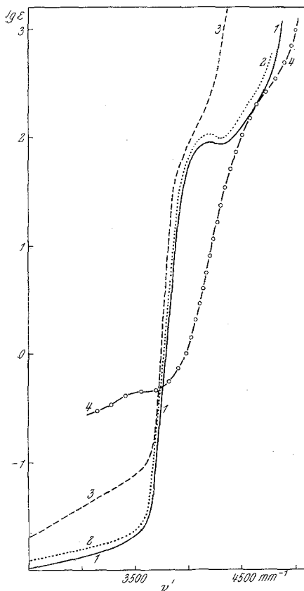
Abb. 3. UV-Spektren von:
